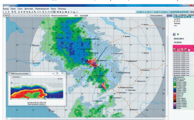
Грозоградный процесс. Данные ДМРЛ-С, 29.04.14.
